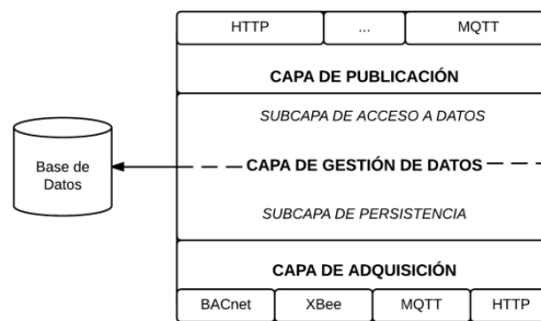
Fig. 1. Arquitectura del sistema
